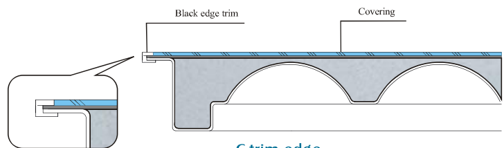
C-trim edge
